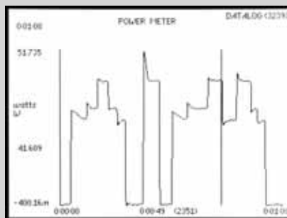
瓦特曲线及游标指出第 2351 记录
