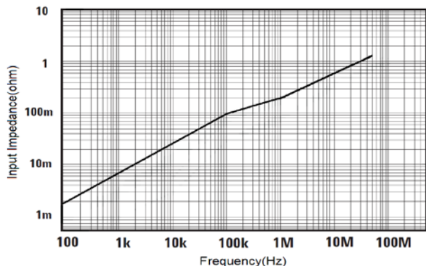
图 6 CP8050A 输入阻抗 VS 频率曲线
