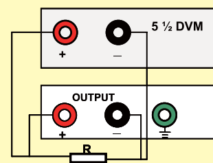
毫欧表接线图
