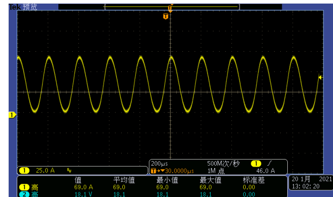
5kHz正弦波
