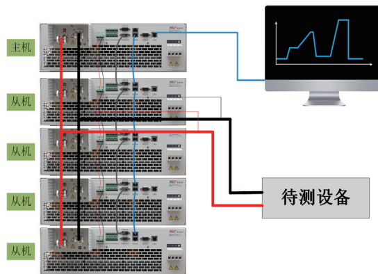
▲ N3300并机运行接线示意图
