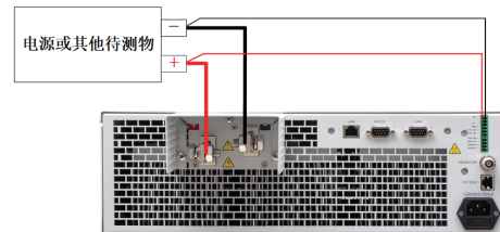
▲ 远端采样连线
