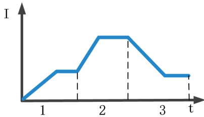
▲ 自动测试波形
