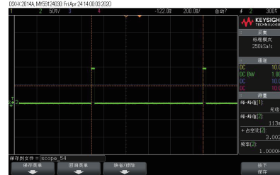
▲ 1Hz 3%占空比电流输出波形
