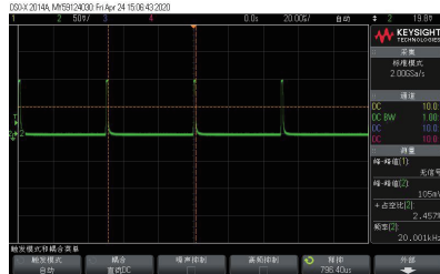
▲ 20kHz 3%占空比电流输出波形
