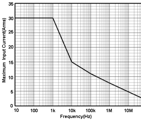
图 2.a HCP0030A 最大测量电流 VS 频率曲线
