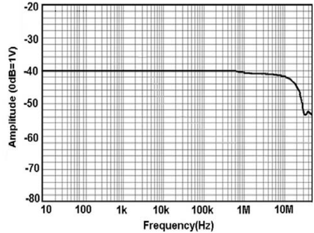
图 7 HCP0150A 幅频曲线
