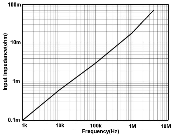
图 12 HCP0300D 输入阻抗 VS 频率曲线
