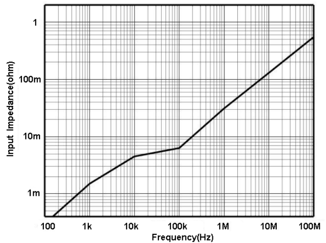
图 3.b HCP0030H 输入阻抗 VS 频率曲线
