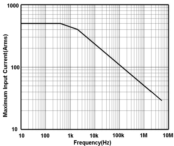
图 14 HCP0500A 最大测量电流 VS 频率曲线 (超过该曲线所示最大电流连续使用会导致探头烧毁)
