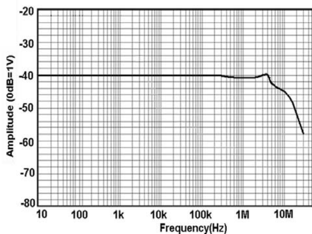
图 13 HCP0500A 幅频曲线
