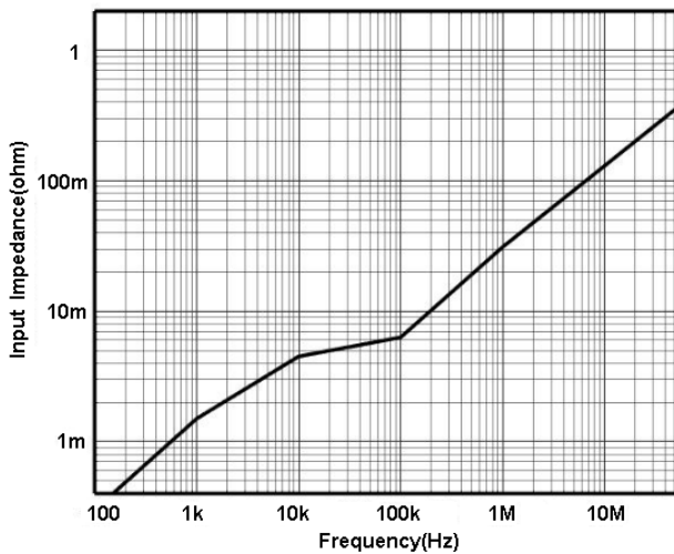
图 3.a HCP0030A 输入阻抗 VS 频率曲线
