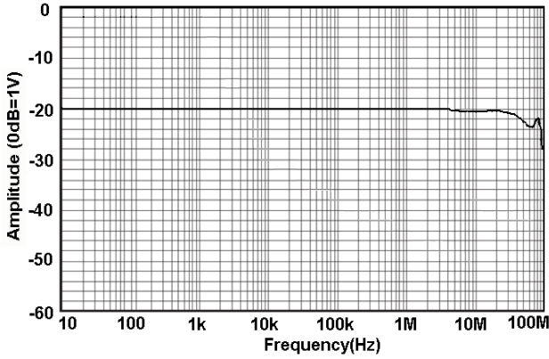
图 1.a HCP0030A 幅频曲线
