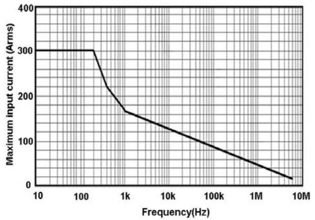
图 11 HCP0300D 最大测量电流 VS 频率曲线 (超过该曲线所示最大电流连续使用会导致探头烧毁)
