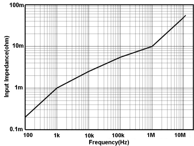
图 9 HCP0150A 输入阻抗 VS 频率曲线
