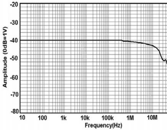
图 10 HCP0300D 幅频曲线
