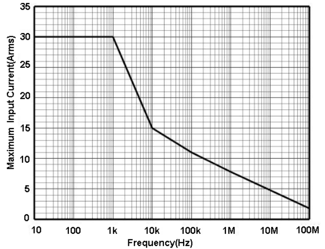
图 2.b HCP0030H 最大测量电流 VS 频率曲线
