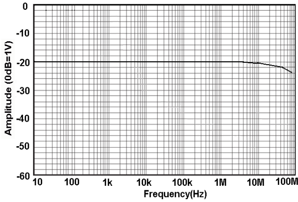
图 4 HCP0050A 幅频曲线
