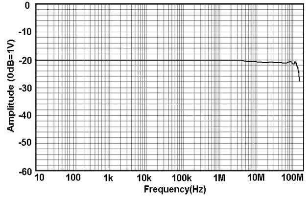
图 1.b HCP0030H 幅频曲线
