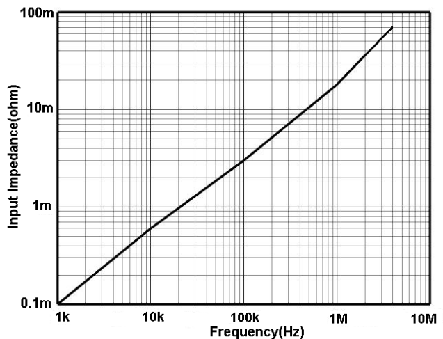
图 15 HCP0500A 输入阻抗 VS 频率曲线
