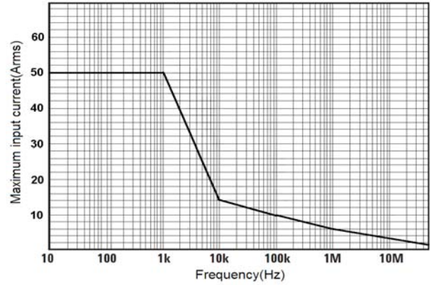
图 5 HCP0050A 最大测量电流 VS 频率曲线 (超过该曲线所示最大电流连续使用会导致探头烧毁)
