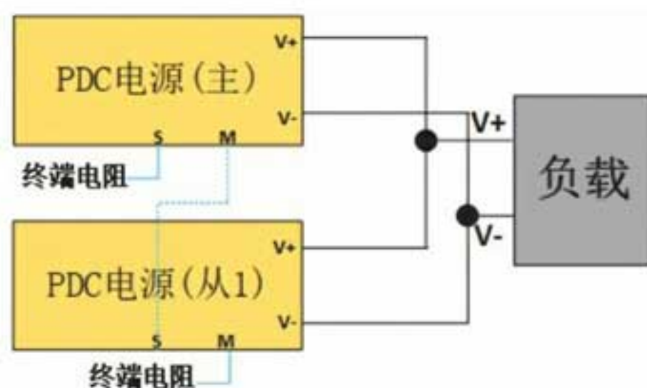
主从并联
