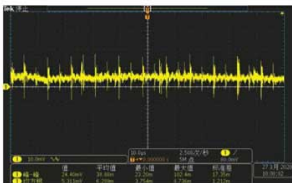
0806S: 80V空载电压纹波
