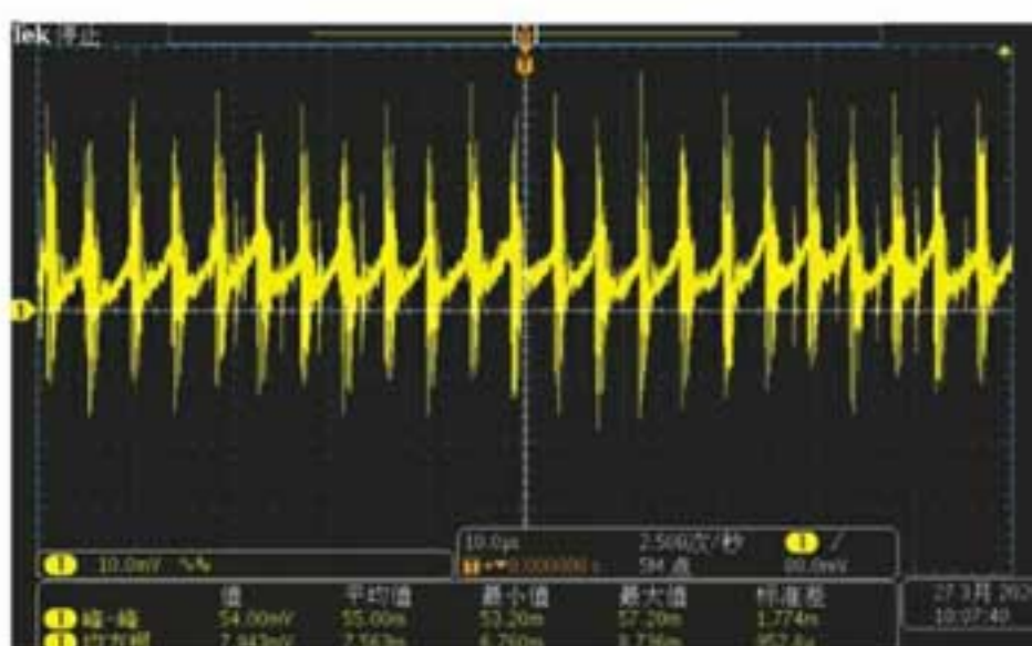
0806S: 80V满载电压纹波
