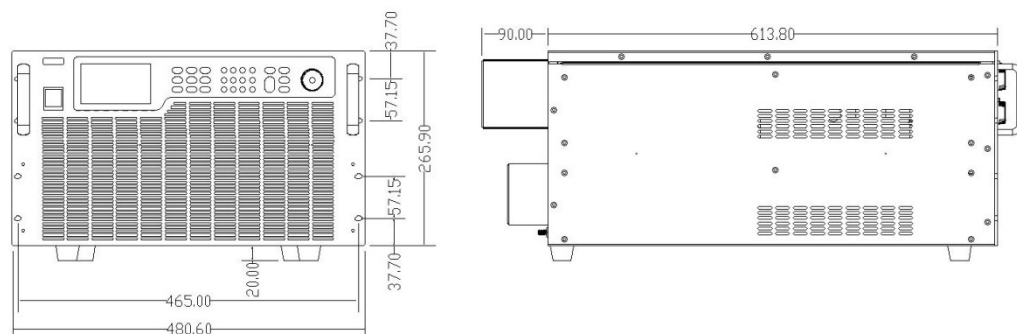
28kW~60kW机型尺寸图（40V及以下机型）
