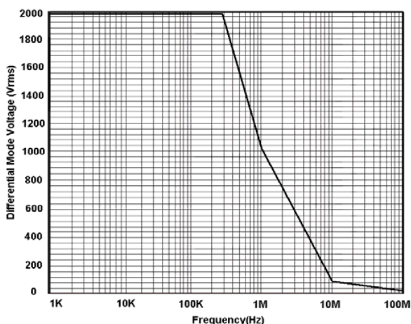
图 3: VP5208A 最大差模电压 VS 频率
