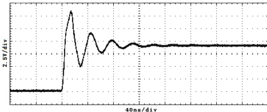
添加输入延长线(CK-301)的波形
