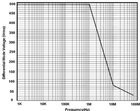
图 1: VP5065A 最大差模电压 VS 频率
