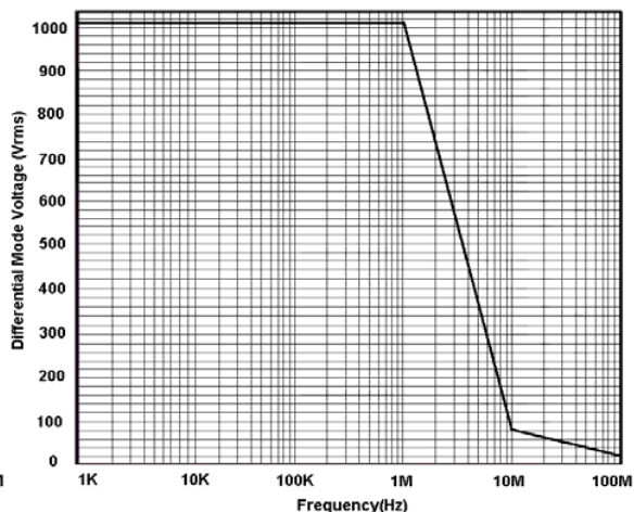
图 2: VP5200A、VP5205A/B 最大差模电压 VS 频率
