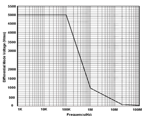
图 4: VP5210A、VP5215A 最大差模电压 VS 频率
