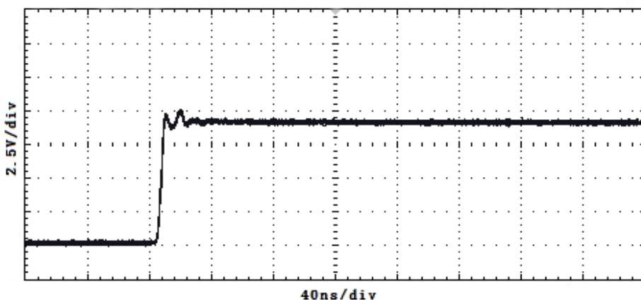
未添加输入延长线的波形
