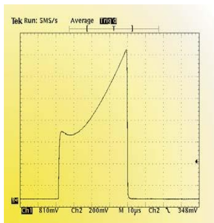
CWT15 测量一个 40\mu\text{s} 脉冲电流 (从 2700A 上升 6700A)
