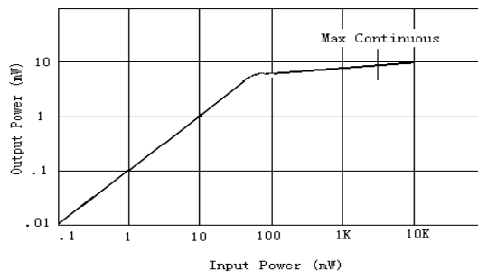
图 2 限幅特性曲线
