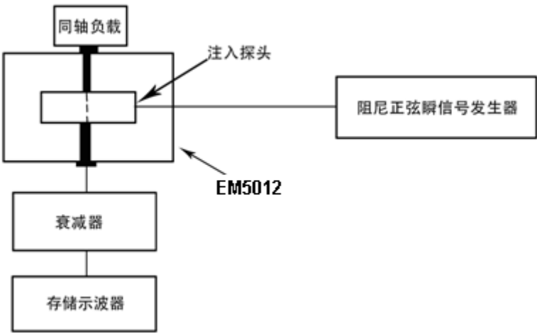
✧ GJB152A-97 中 CS116 电流探头校准图
