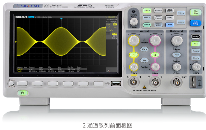
2 通道系列前面板图
