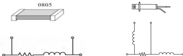
普通电阻和同轴分流器的等效电路图
