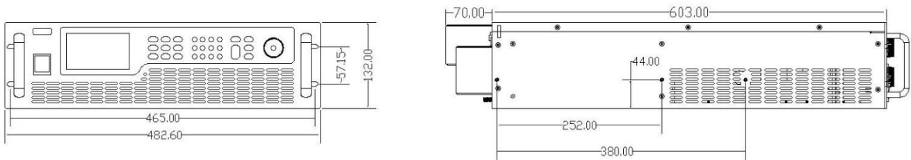
5kW~15kW机型尺寸图（40V及以上机型）
