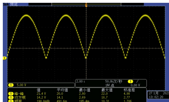
序列功能生成的半波正弦
