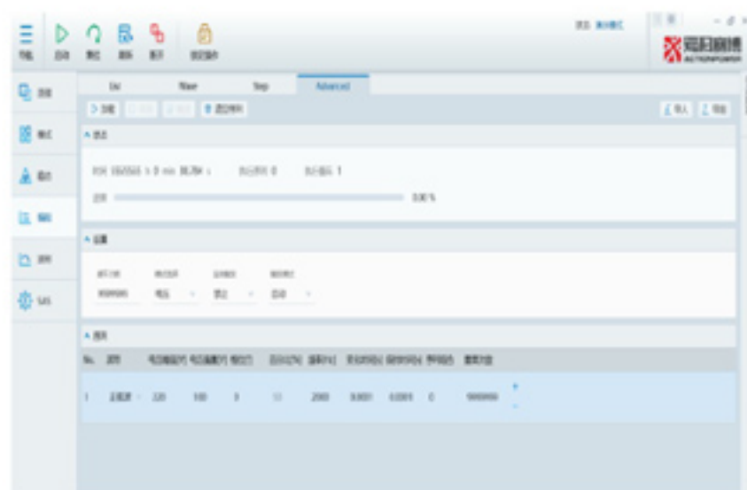
叠加2000Hz正弦波编程界面
