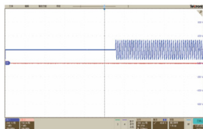
DC200V叠加AC100V正弦波
