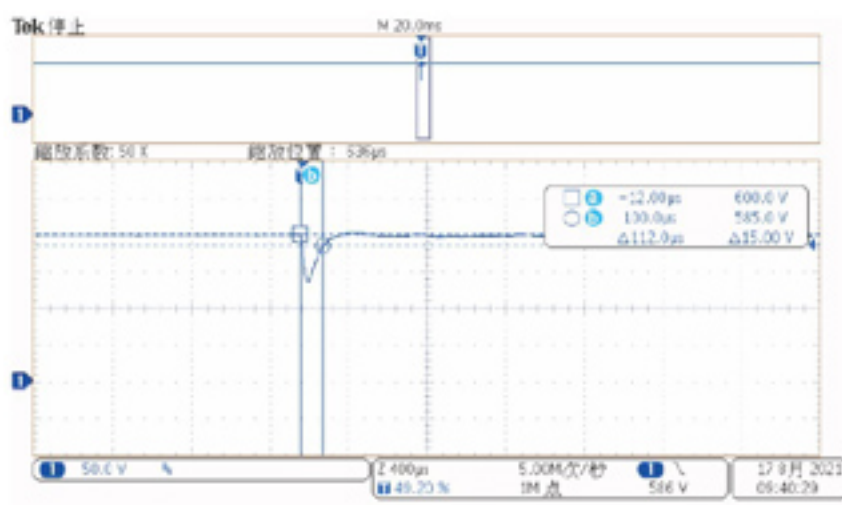
40%-90%负载突加输出电压响应时间
