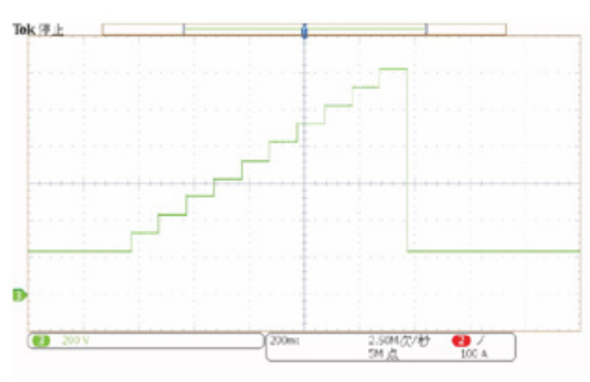
编程波形示例
