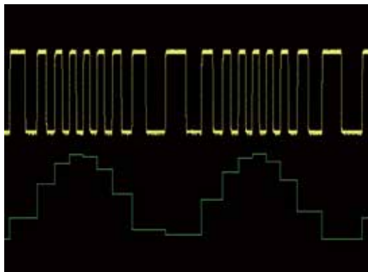
编码器脉冲信号的F-V转换
