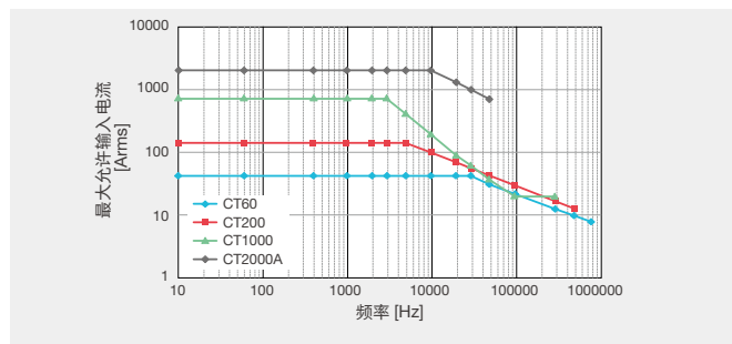
CT系列一次电流减额特性 (例) *
