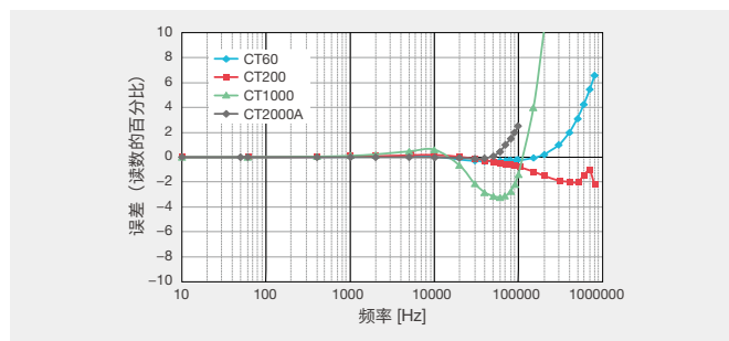
CT系列频率特性 (例) *
