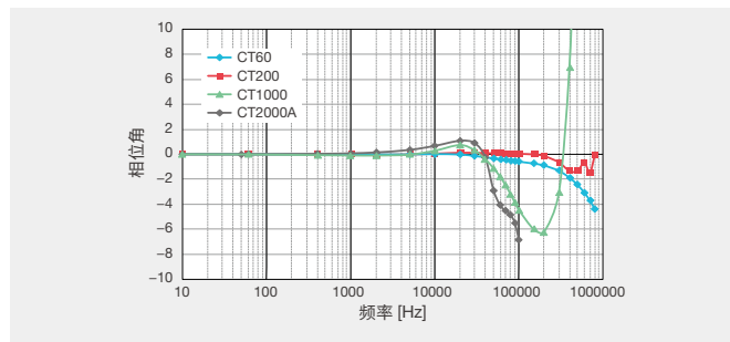
CT系列相位特性 (例) *
