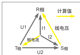
图1 线电压/相电流
