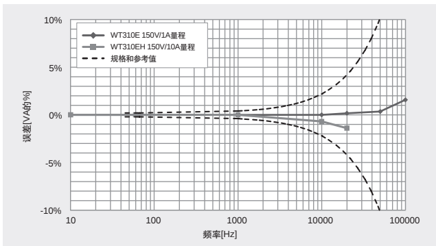
频率与功率精度特性曲线对比示例 ( \cos\theta = 0 时功率规格)
