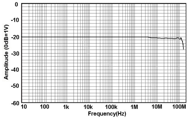
图 1.b CP0030H 幅频曲线
