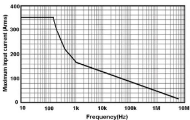
图 11 CP0300A 最大测量电流 VS 频率曲线 (超过该曲线所示最大电流连续使用会导致探头烧毁)
