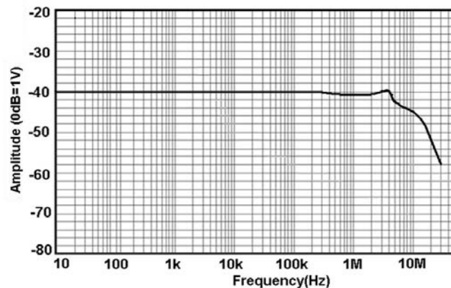
图 13 CP0500A 幅频曲线
