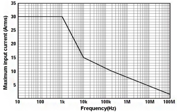
图 3.b CP0030H 输入阻抗 VS 频率曲线
