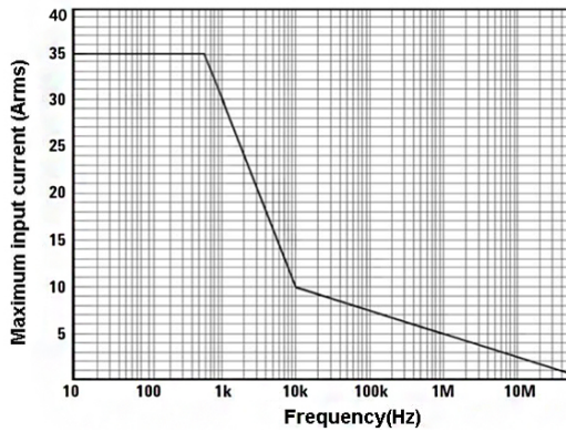
图 3.a CP0030A 输入阻抗 VS 频率曲线
