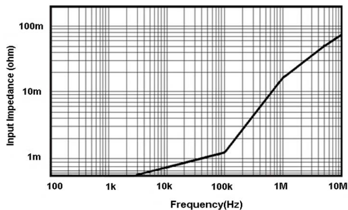
图 15 CP0500A 输入阻抗 VS 频率曲线
