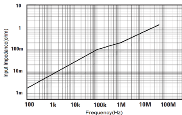
图 6 CP0050A 输入阻抗 VS 频率曲线
