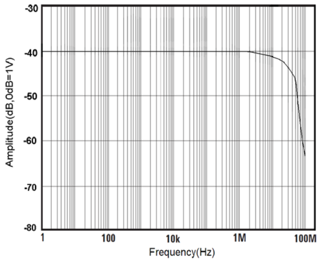
图 12 CP303 幅频曲线
