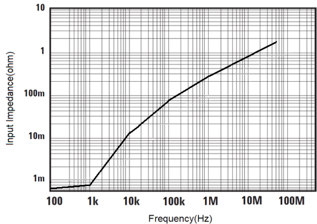
图 19 CP305 插入损耗 VS 频率曲线
