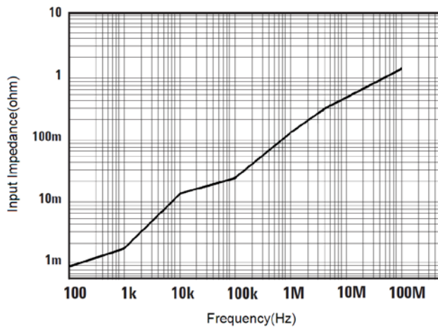
图 20 CP303 插入损耗 VS 频率曲线
