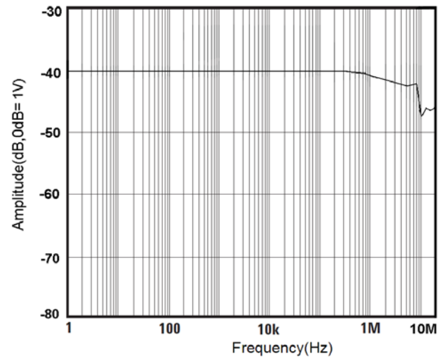
图 13 CP404XL 幅频曲线
