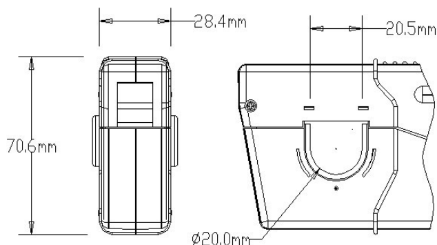
图 9 CP303 和 CP404XL 钳口尺寸图
