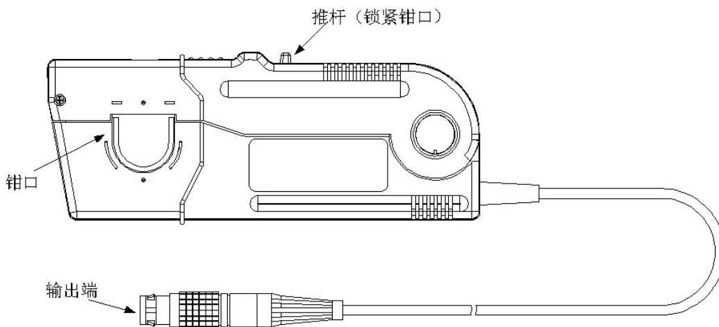
图 4：CP303 和 CP404XL 结构图
