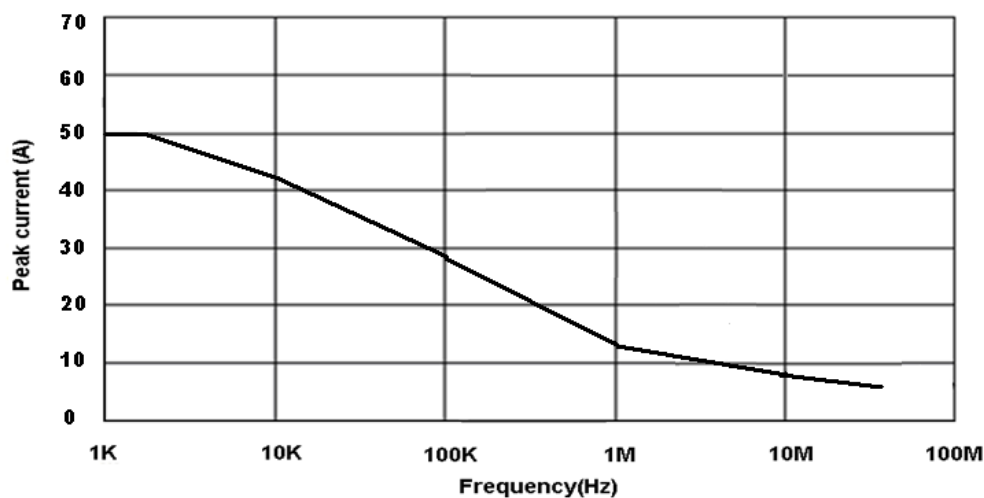
图 15 CP305 最大峰值电流 VS 频率曲线 (超过该曲线所示最大电流连续使用会导致探头烧毁)
