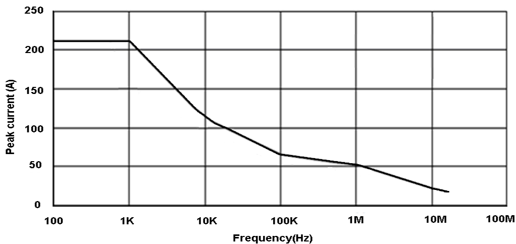
图 16 CP303 最大峰值电流 VS 频率曲线 (超过该曲线所示最大电流连续使用会导致探头烧毁)
