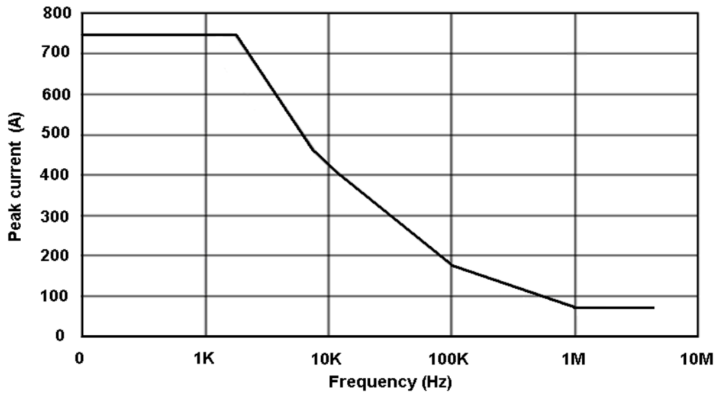
图 17 CP404XL 最大峰值电流 VS 频率曲线 (超过该曲线所示最大电流连续使用会导致探头烧毁)
