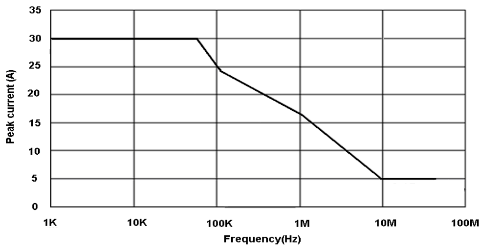
图 14 CP312 最大峰值电流 VS 频率曲线 (超过该曲线所示最大电流连续使用会导致探头烧毁)
