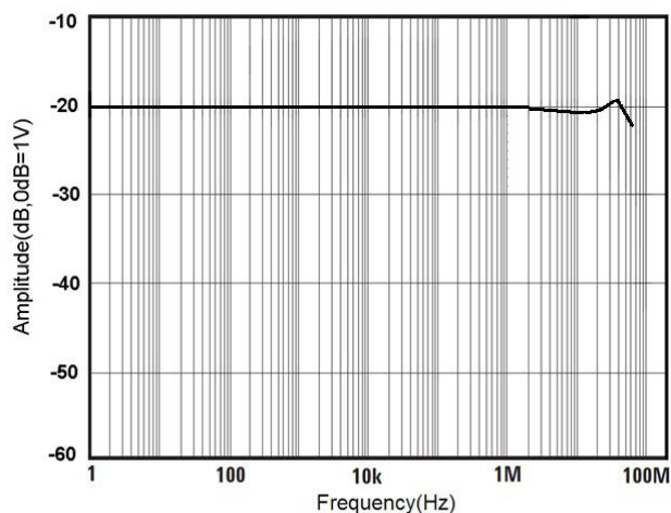
图 11 CP305 幅频曲线
