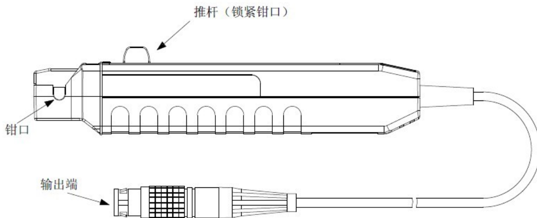
图 3：CP312 和 CP305 结构图
