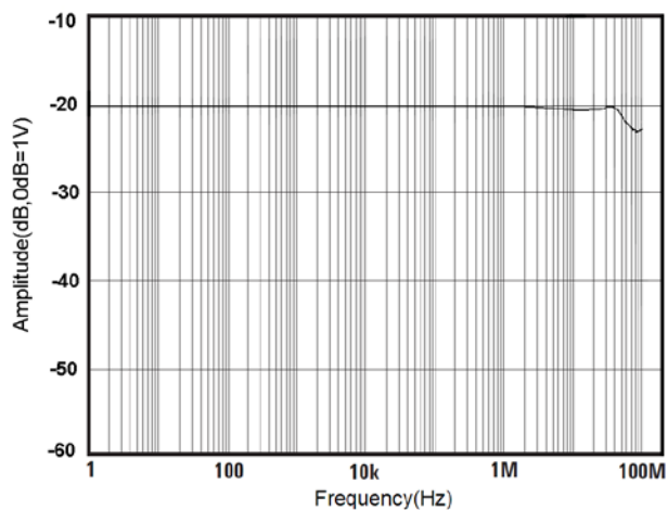
图 10 CP312 幅频曲线
