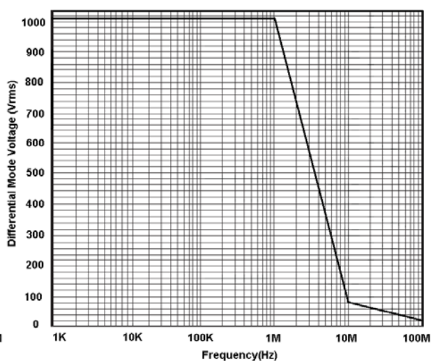
图 2: DP6150 (A/B) 最大差模电压 VS 频率
