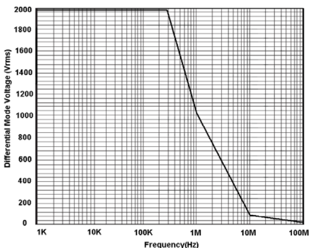
图 3: DP6280 最大差模电压 VS 频率
