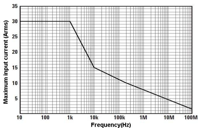
图 2.b CP00030H 最大测量电流 VS 频率曲线 (超过该曲线所示最大电流连续使用会导致探头烧毁)
