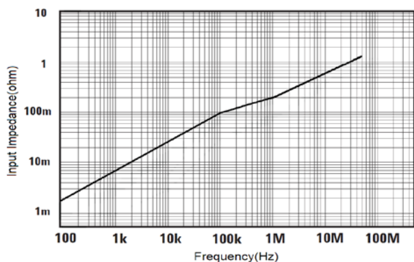
图 6 CP0050A 输入阻抗 VS 频率曲线
