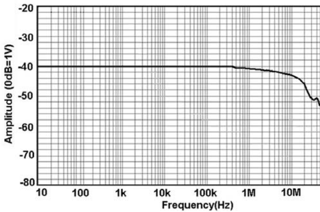
图 10 CP0300A 幅频曲线
