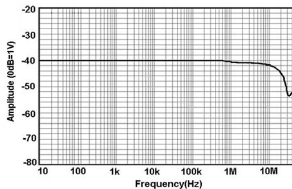
图 7 CP0150A 幅频曲线
