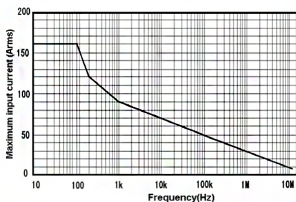
图 8 CP0150A 最大测量电流 VS 频率曲线 (超过该曲线所示最大电流连续使用会导致探头烧毁)
