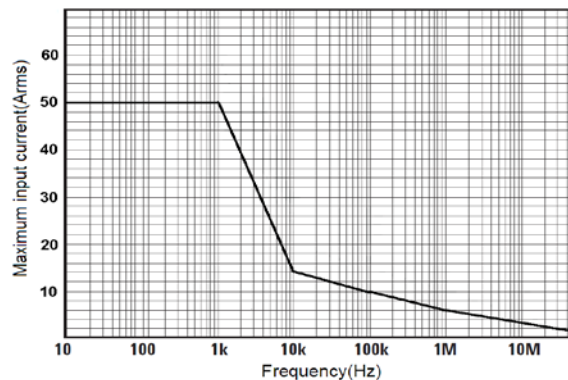
图 5 CP0050A 最大测量电流 VS 频率曲线 (超过该曲线所示最大电流连续使用会导致探头烧毁)
