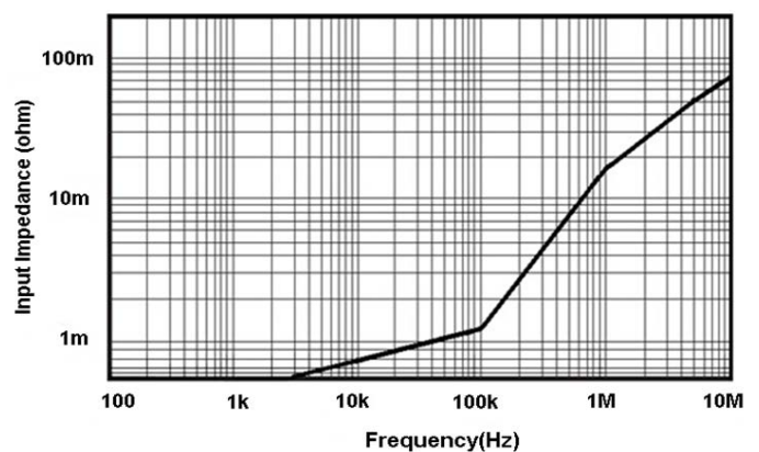
图 15 CP0500A 输入阻抗 VS 频率曲线
