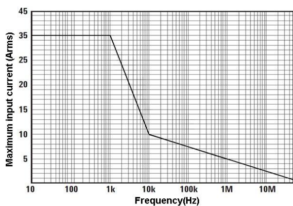
图 2.a CP00030A 最大测量电流 VS 频率曲线 (超过该曲线所示最大电流连续使用会导致探头烧毁)
