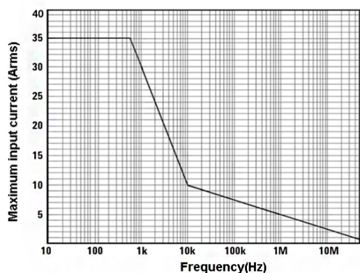
图 3.a CP00030A 输入阻抗 VS 频率曲线
