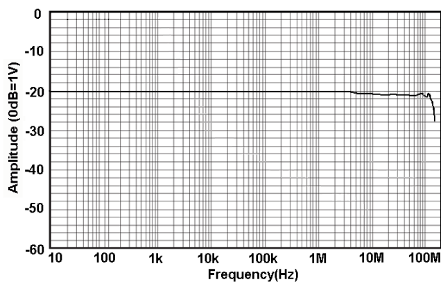
图 1.b CP00030H 幅频曲线
