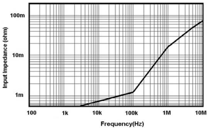
图 12 CP0300A 输入阻抗 VS 频率曲线
