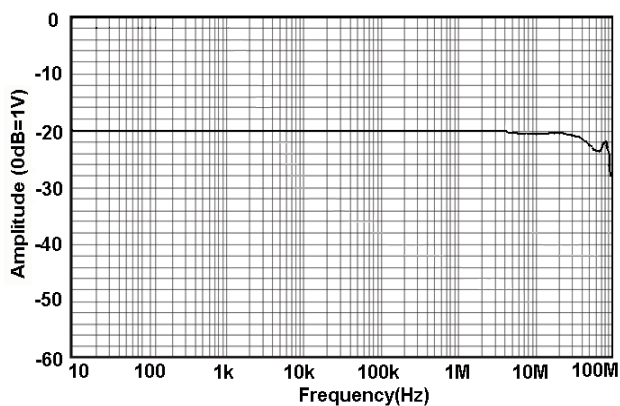
图 1.a CP00030A 幅频曲线
