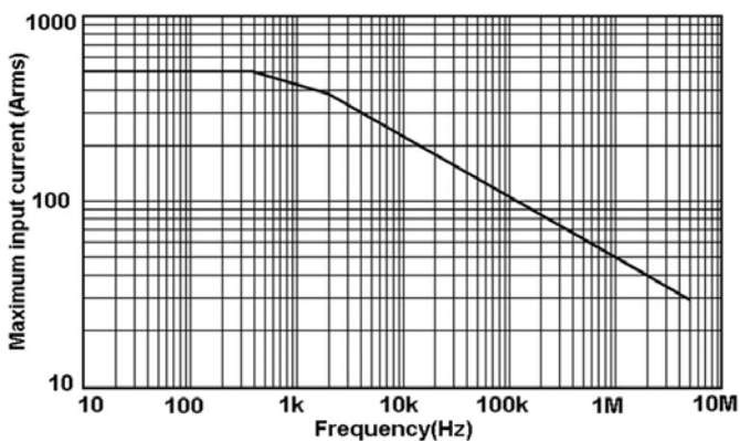
图 14 CP0500A 最大测量电流 VS 频率曲线 (超过该曲线所示最大电流连续使用会导致探头烧毁)
