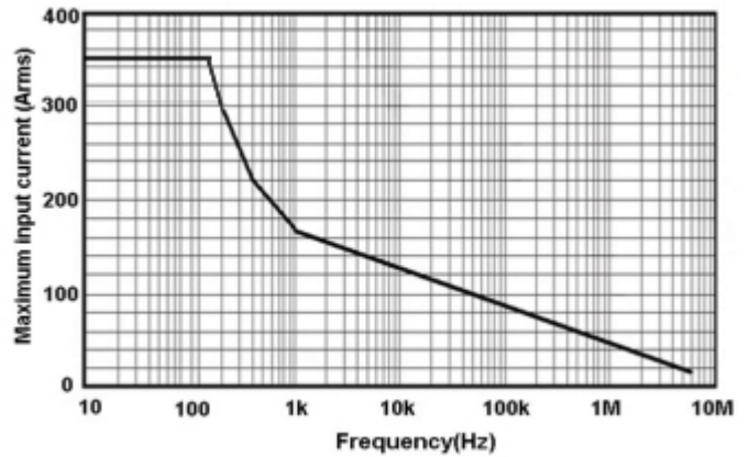
图 11 CP0300A 最大测量电流 VS 频率曲线 (超过该曲线所示最大电流连续使用会导致探头烧毁)
