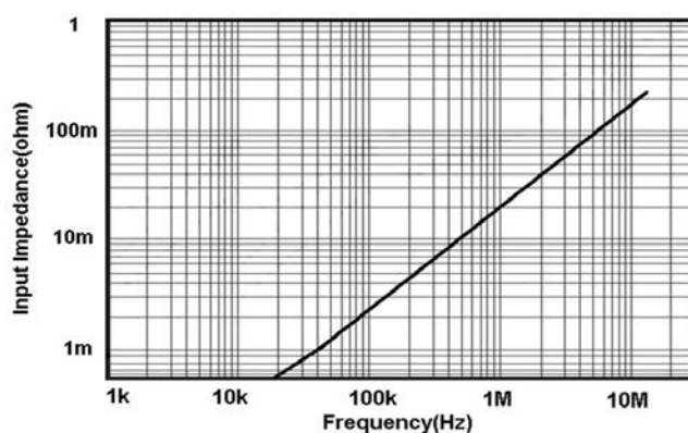
图 9 CP0150A 输入阻抗 VS 频率曲线
