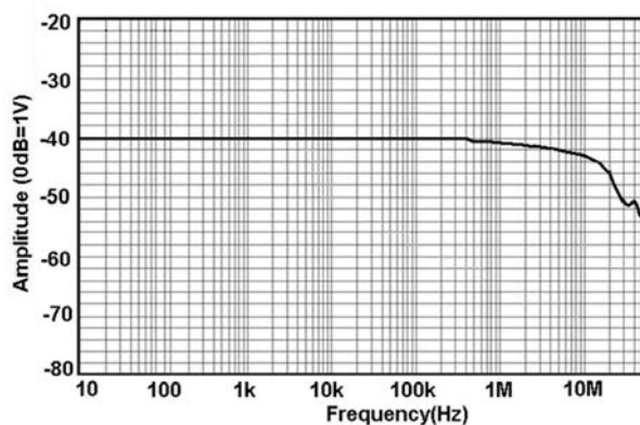
图 10 CP8300A 幅频曲线
