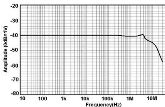
图 13 CP8500A 幅频曲线
