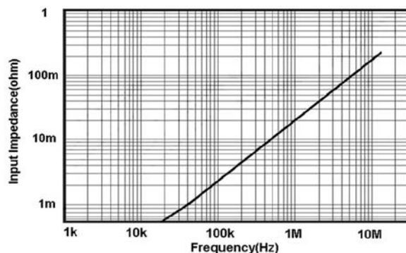
图 9 CP8150A 输入阻抗 VS 频率曲线
