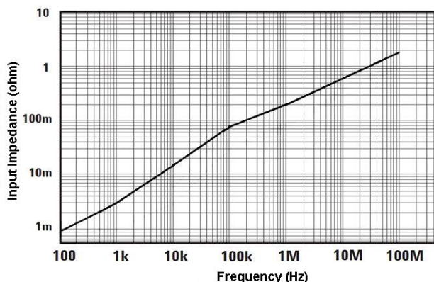
图 3. b CP8030H 输入阻抗 VS 频率曲线
