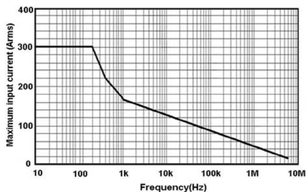
图 11 CP8300A 最大测量电流 VS 频率曲线 (超过该曲线所示最大电流连续使用会导致探头烧毁)
