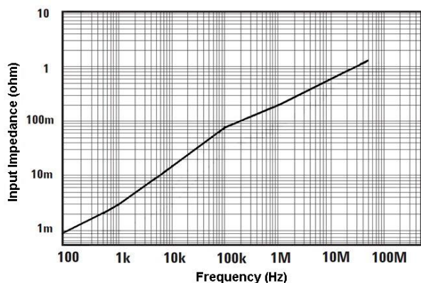
图 3. a CP8030B 输入阻抗 VS 频率曲线
