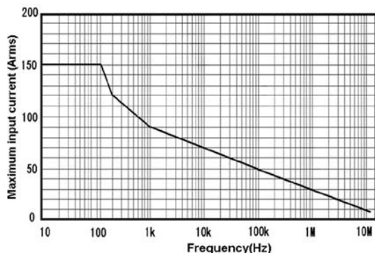
图 8 CP8150A 最大测量电流 VS 频率曲线 (超过该曲线所示最大电流连续使用会导致探头烧毁)
