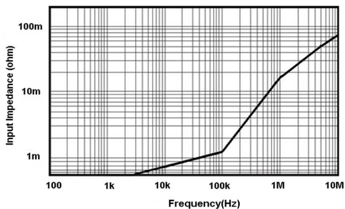
图 15 CP8500A 输入阻抗 VS 频率曲线
