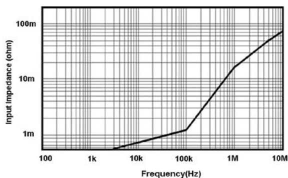
图 12 CP8300A 输入阻抗 VS 频率曲线
