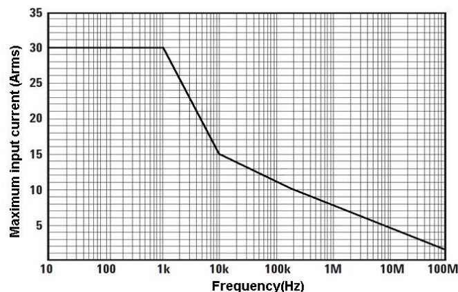
图 2. b CP8030H 最大测量电流 VS 频率曲线 (超过该曲线所示最大电流连续使用会导致探头烧毁)
