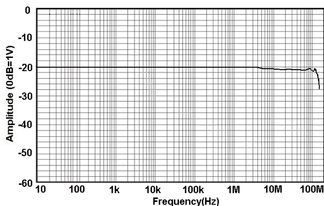
图 1 . b CP8030H 幅频曲线
