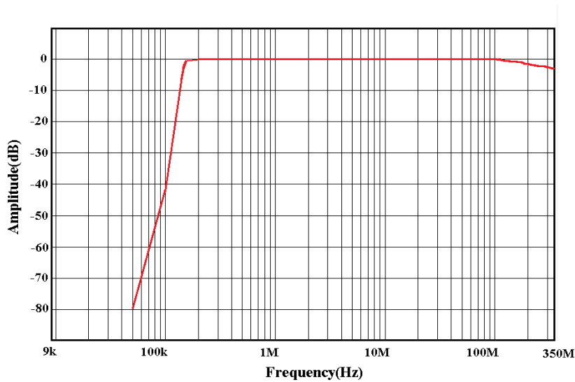
图 1 频响曲线
