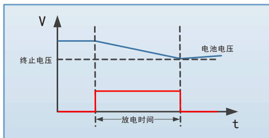
容量测试时电压与电流曲线
