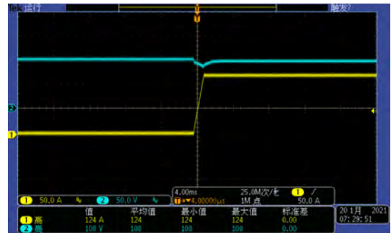
FT68206E-150-600额定6kW，瞬间带载12kW
